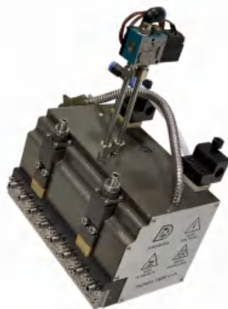
200mm欧米茄纤维喷枪 XD-25XW200mm
