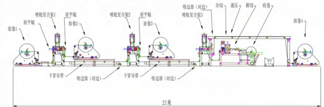
俊鼎达-1600 3喷胶4层布熔喷复合机-整体方案2 2021/12/01
