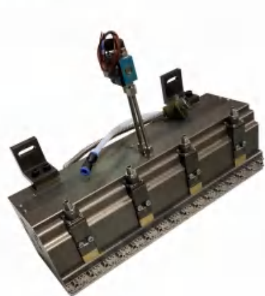
400mm欧米茄纤维喷枪 XD-25XW400mm
